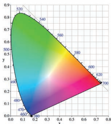
Illustrasjon 19: CIEs fargediatram. Det synlige fargespekteret er visualisert, linjen som omgir fargefeltet angir bølgelengdene i nanometer.
