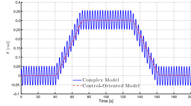
(d) The orientation of the robot
