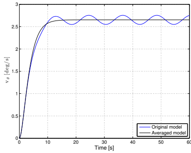
(d) The angular velocity, v_\theta
